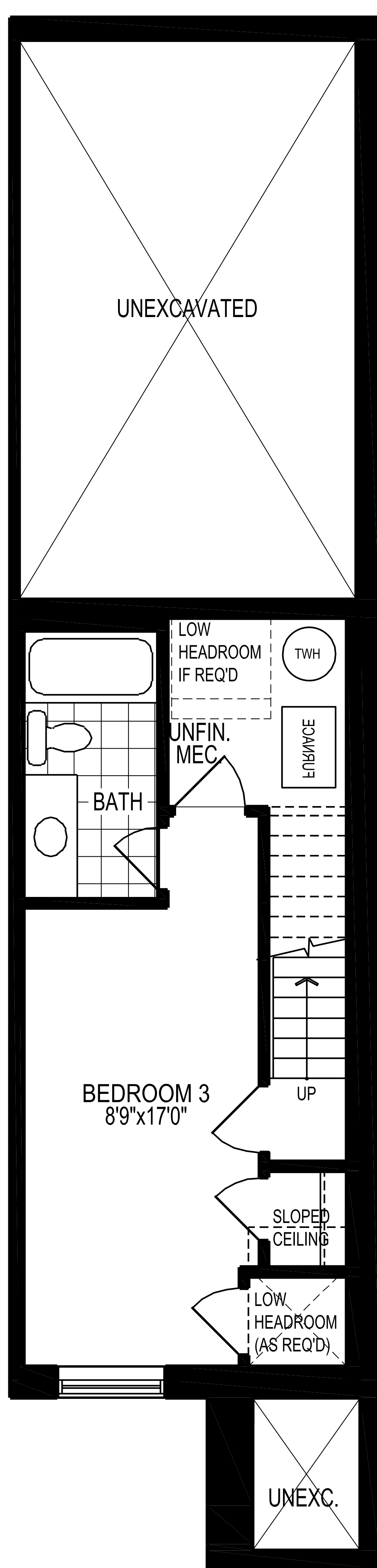
BASEMENT PLAN 'A' & 'B'
